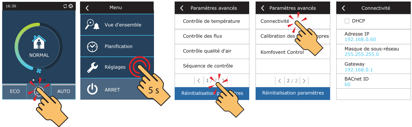
Fig. 18. Visualiser et modifier l'adresse IP de la centrale de traitement d'air depuis le panneau de commande
