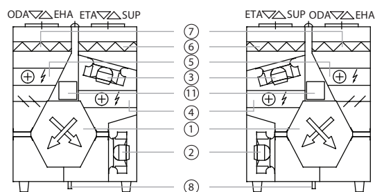
CÔTÉ D'INSPECTION À DROITE
