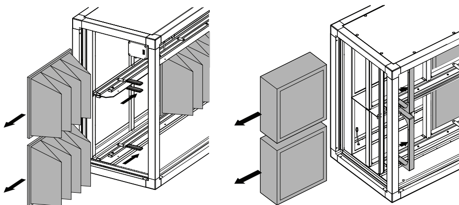
Fig. 4 Dispositif de fixation du filtre
