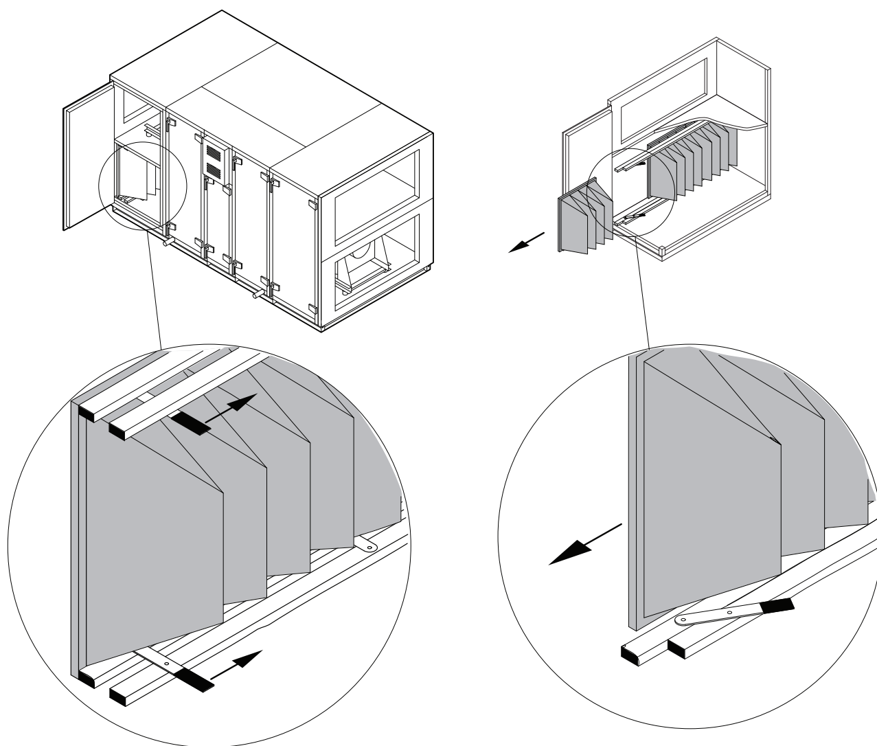
Fig. 3. Dispositif de fixation du filtre
