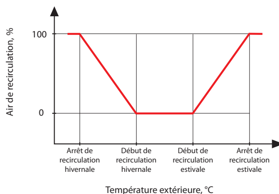
Fig. 2. Fonctionnement de la fonction REC
