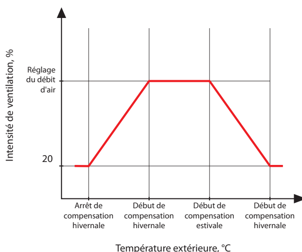
Fig. 1. Fonctionnement de la fonction OCV
