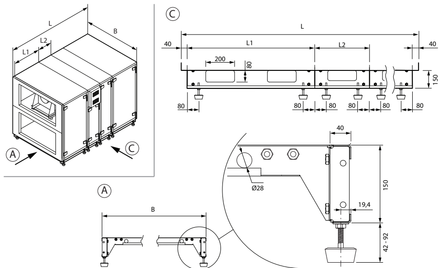
Fig. 17. Cadre d'installation équipé de pieds réglables
