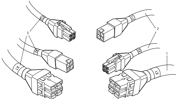
Fig. 50. Raccordement des câbles entre les sections 1 – câble d'alimentation électrique, 2 – câbles de communication entre les cartes de circuits imprimés, 3 – étiquettes avec numéros de connexion
