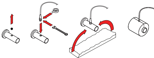
Fig. 27. Installation d'une sonde de température de l'eau de retour avec filetage 3
