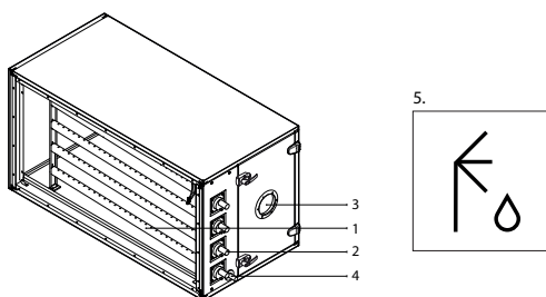
Fig. 10. Section Humidificateur 1 – distributeurs de vapeur, 2 – tuyaux de connexion de flexible de vapeur, 3 – fenêtre d'inspection, 4 – tuyau d'évacuation des condensats, 5 – Étiquette de la section Humidificateur
