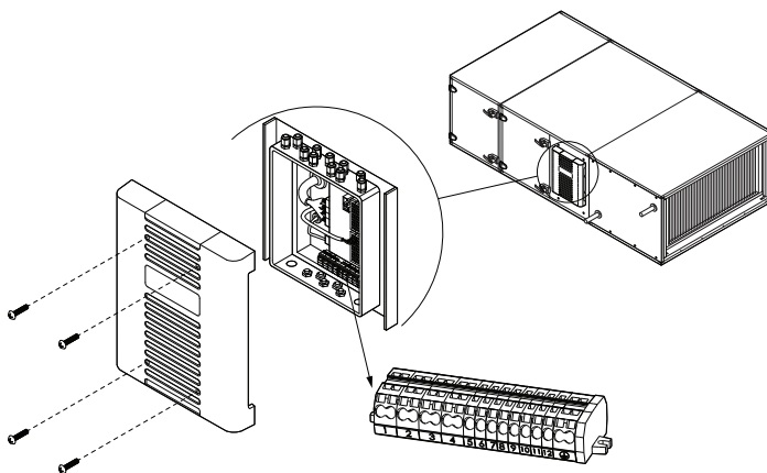
Fig. 46. Bornes de raccordement des centrales de traitement d'air VERSO RA
