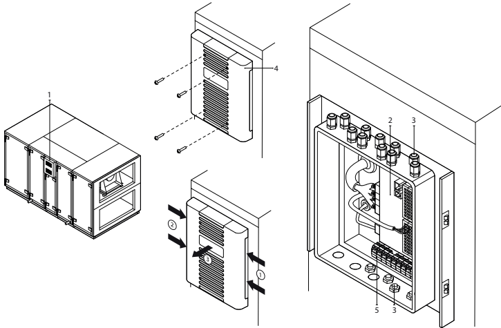
Fig. 37. Boîtier d'automatisation
