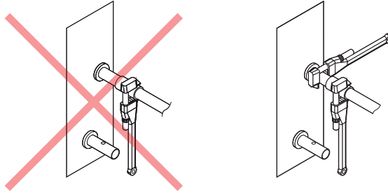
Fig. 25. Connexion des manchons
