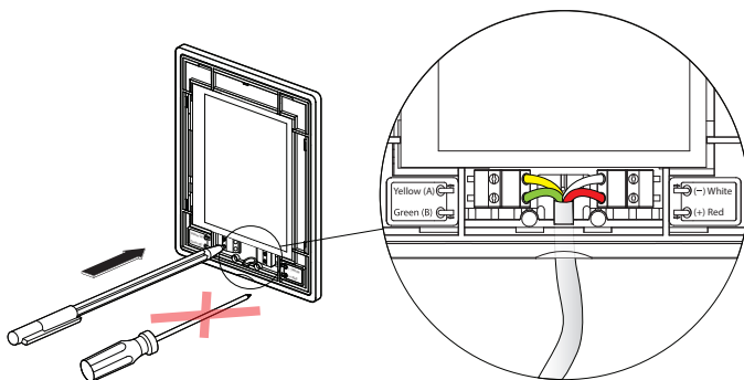
Fig. 49. Câblage du panneau de commande
