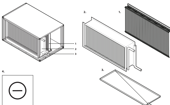
Fig. 6. Section de refroidisseur 1 – éliminateur de gouttes, 2 – bobine d'eau/réfrigérant 3 – bac de condensation, 4 – étiquette de la section de refroidisseur
