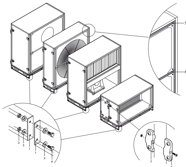
Fig. 21. Raccordement externe et scellement des sections
