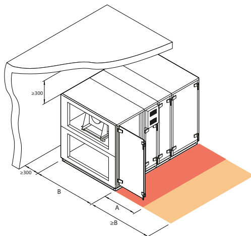
Fig. 18. Zone d'inspection de l'unité
