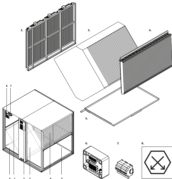
Fig. 2. Section d'échangeur de chaleur à contre-courant (CF)
