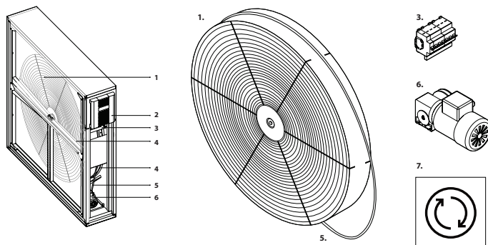
Fig. 3. Section du récupérateur rotatif
