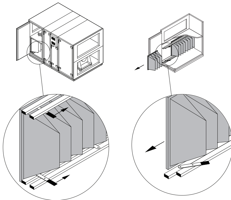
Fig. 55. Dispositif de fixation du filtre
