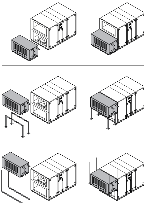
Fig. 24. Exemples d'installations de section chauffage/refroidissement
