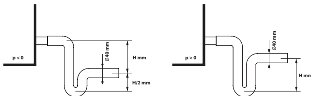
Fig. 28. Installation d'un siphon sans vanne unidirectionnelle
