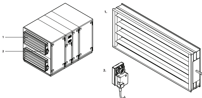
Fig. 8. Registre de fermeture d'air
