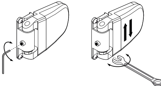
Fig. 20. Réglage des charnières
