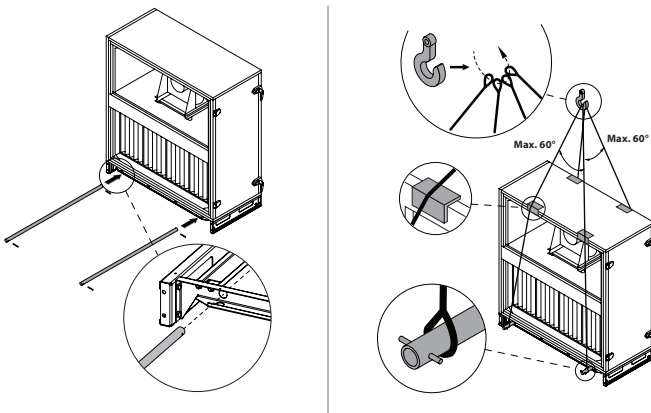
Fig. 14. Levage des sections individuelles 1
