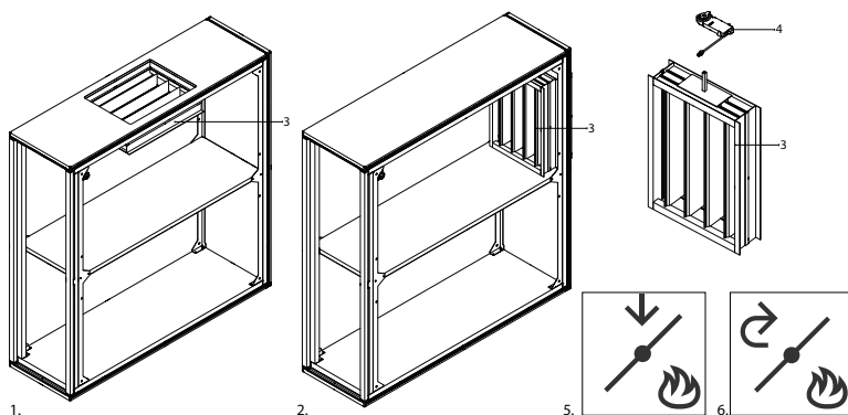
Fig. 11. Section d'extraction de la fumée
