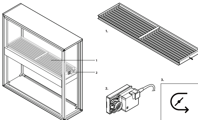
Fig. 5. Section recirculation 1 – registre de mélange d'air, 2 – actionneur de registre, 3 – étiquette de la section recirculation
