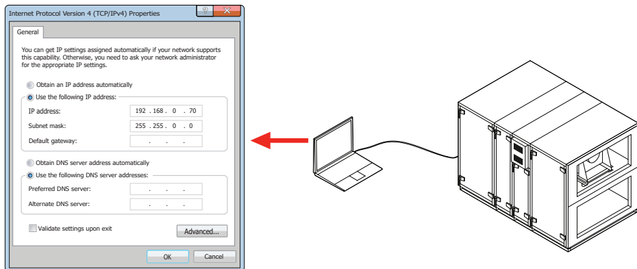
Fig. 53. Paramètres du réseau informatique pour une connexion directe à l'unité
