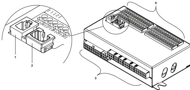
Fig. 38. Carte mère du panneau de commande C5
