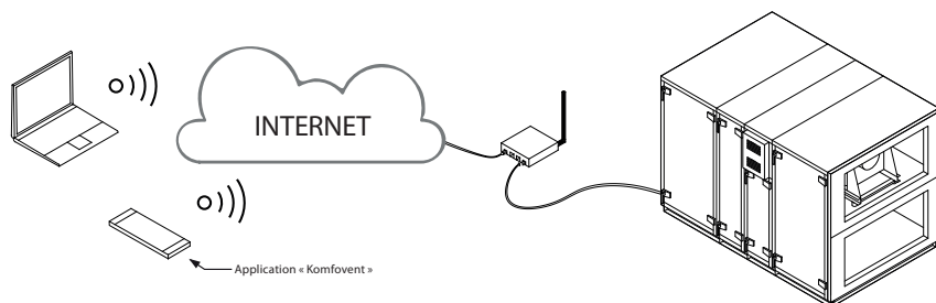
Fig. 54. Exemples de connexion des unités de traitement de l'air à l'Internet ou au réseau local
