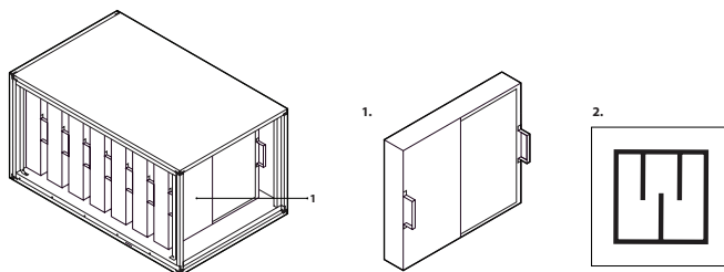
Fig. 9. Section de suppression du bruit 1 – cloisons d'absorption de bruit amovibles, 2 – étiquette de la section du silencieux
