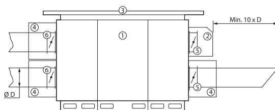
Fig. 33. Accessoires des unités à installer à l'extérieur
