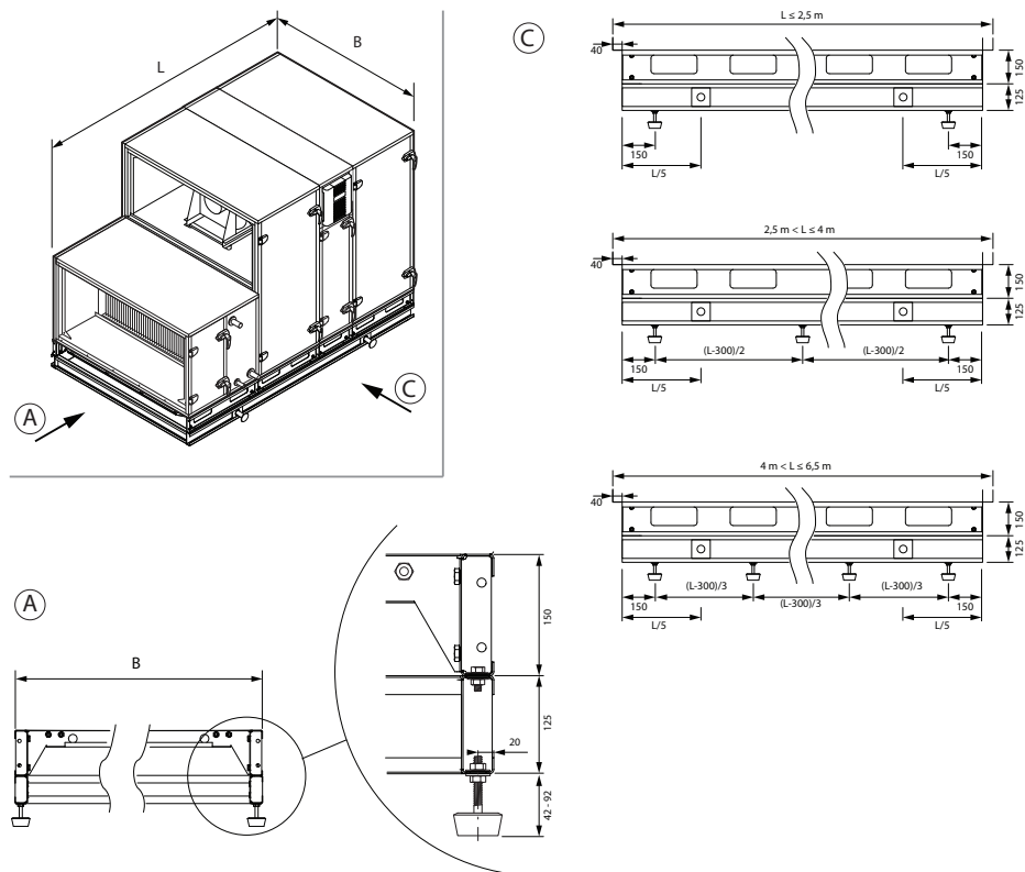
Fig. 16. Dimensions du cadre de montage renforcé
