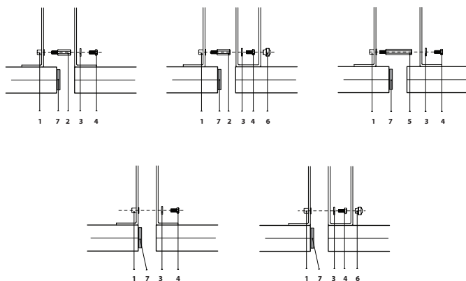
Fig. 22. Types de connexions de la section interne
