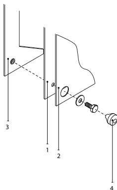
Fig. 23. Raccordement interne dans une section ventilateur 1 – cornière de serrage de la section ventilateur, 2 – mur sur lequel est monté le ventilateur, 3 – Cornière de serrage des autres sections, 4 – œilleton d29
