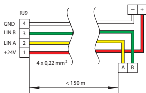
Fig. 48. Schéma de câblage du panneau de commande
