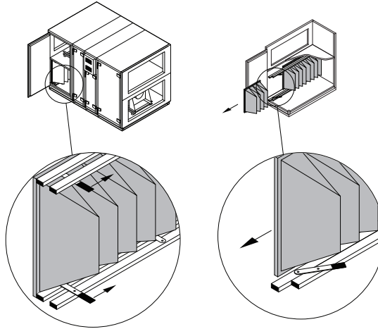
Fig. 4 Dispositif de fixation du filtre
