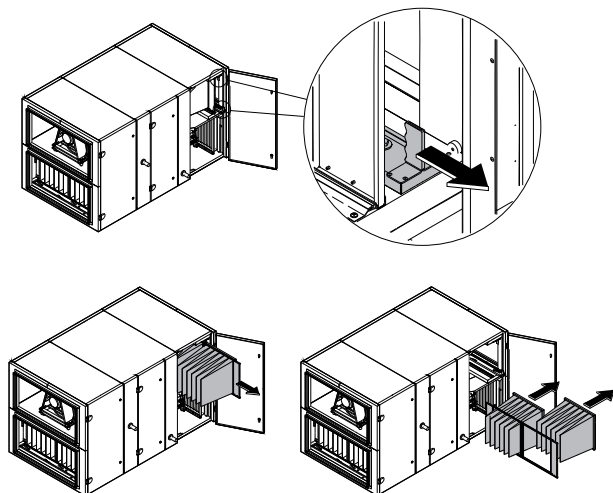
Fig. 3. Dispositif de fixation du filtre
