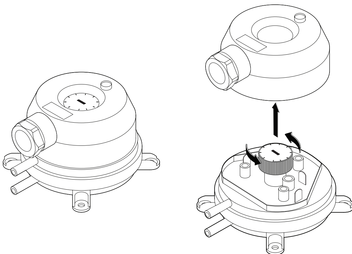
Fig. 2. Pressostat d'air
