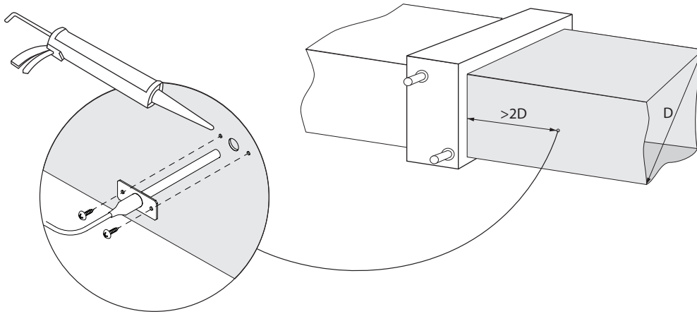
Fig. 21. Installation d'un capteur de température d'air de soufflage
