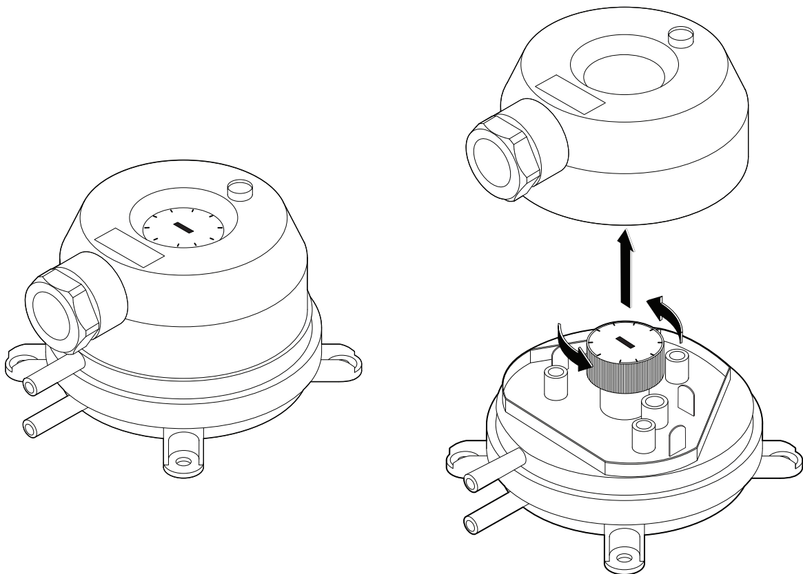
Fig. 28. Pressostat
