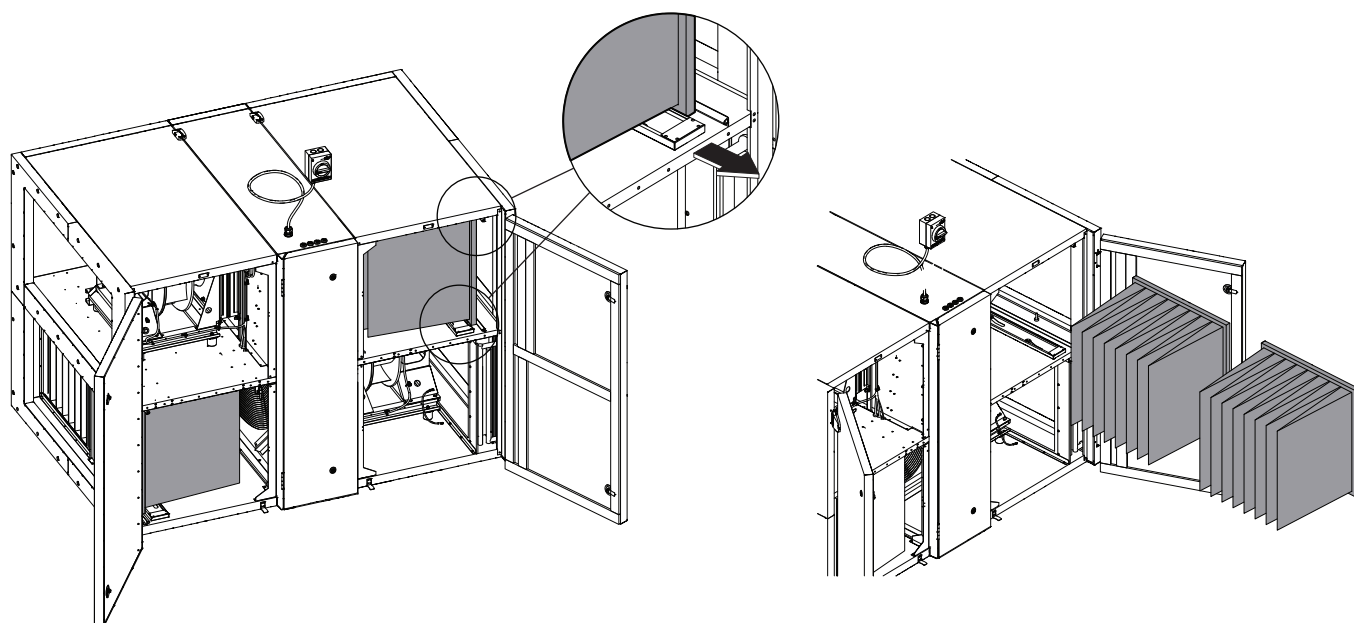
Fig. 29. Un exemple montrant comment remplacer les filtres à poches
