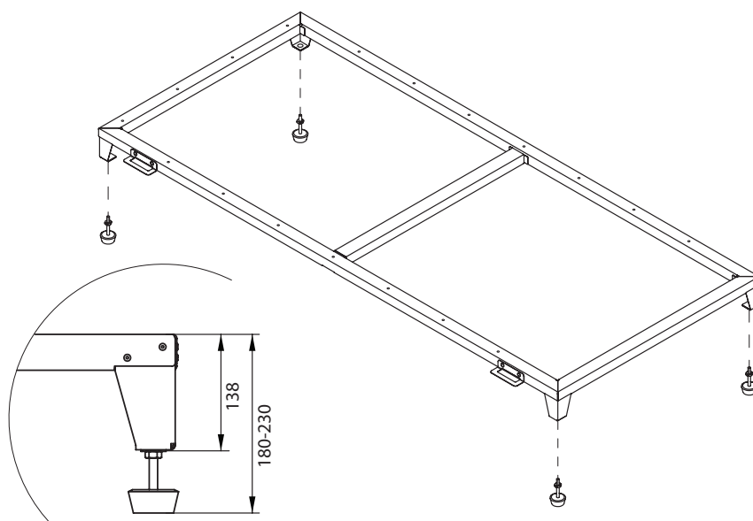
Fig. 6. Cadre de montage de l'unité avec pieds réglables (à commander séparément)
