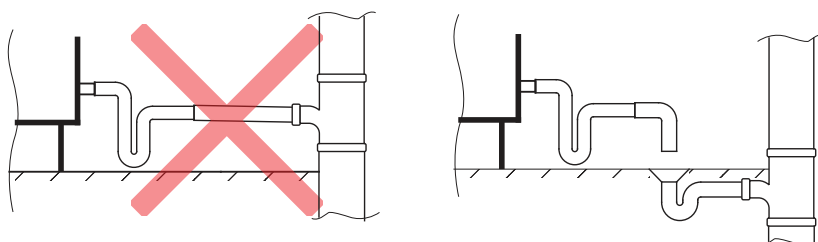
Fig. 15. Raccordement de l'évacuation de la condensation au réseau d'égouts
