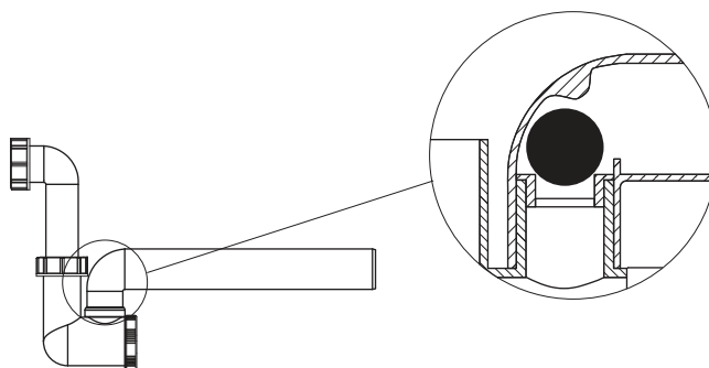
Fig. 14. Exemple d'un siphon avec vanne unidirectionnelle
