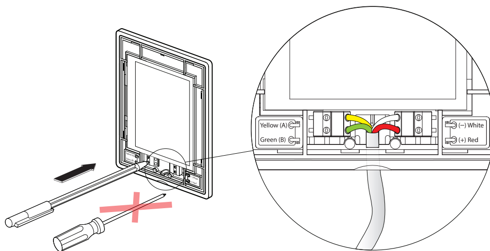
Fig. 23. Câblage du panneau de commande
