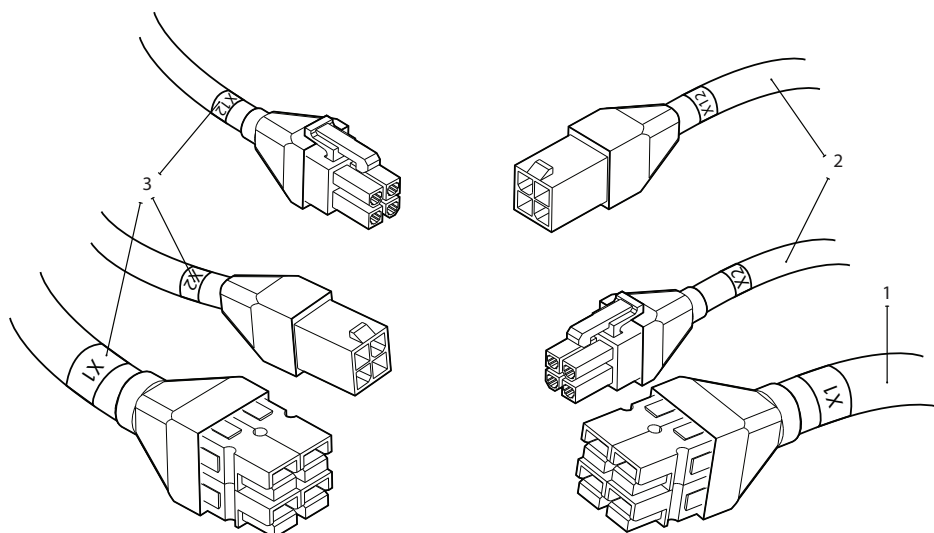
Fig. 24. Raccordement des câbles entre les sections
