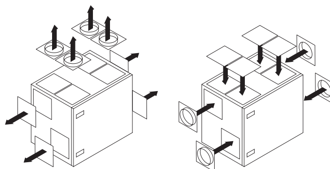
Fig. 2. Déplacement des raccords de conduites des unités universelles
