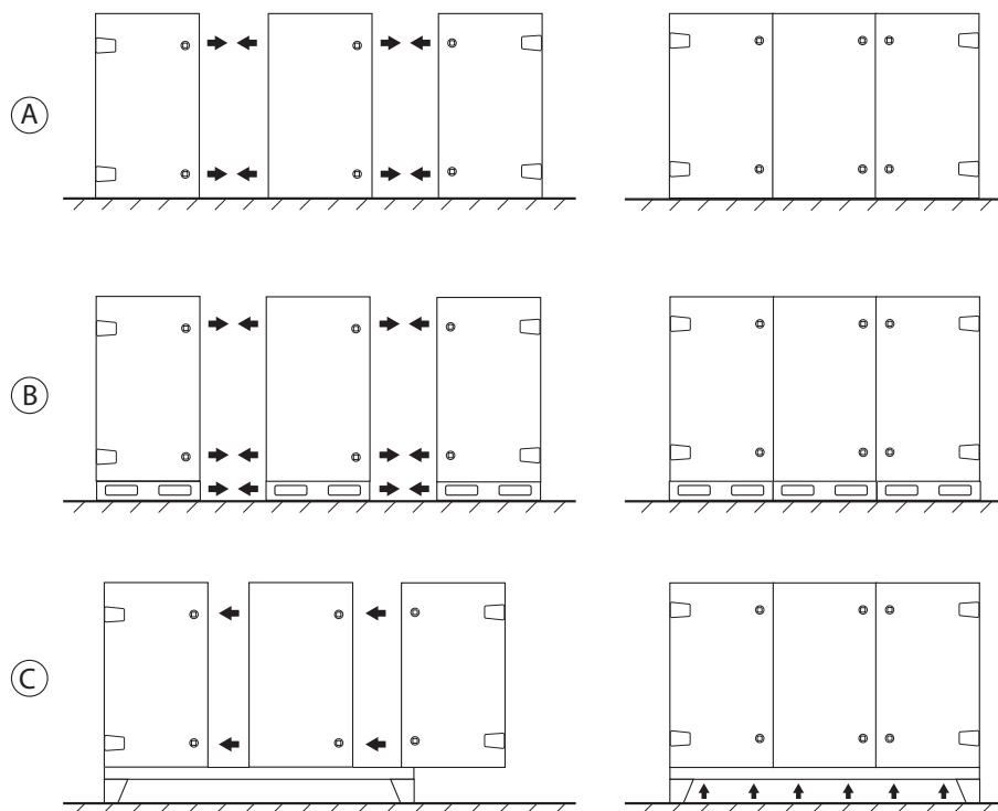
Fig. 9. Raccordement des sections sans le cadre de montage et avec le cadre de montage A – sans cadre de montage, B – avec cadre de montage assemblé en usine pour chaque section distincte, C – avec cadre de montage commandé séparément
