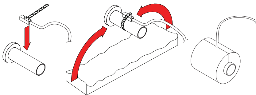
Fig. 12. Installation d'un capteur de température de l'eau de retour
