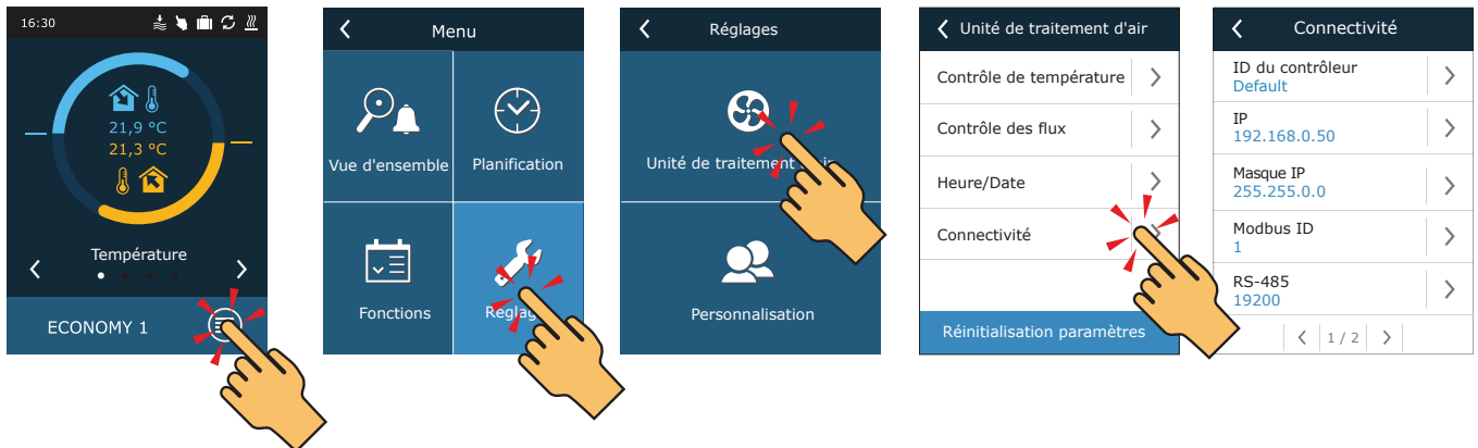
Fig. 25. Visualisation et modification de l'adresse IP à l'aide d'un panneau de commande
