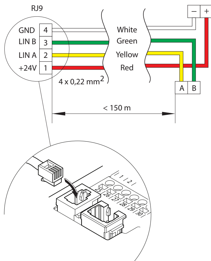
Fig. 22. Schéma de câblage du panneau de commande
