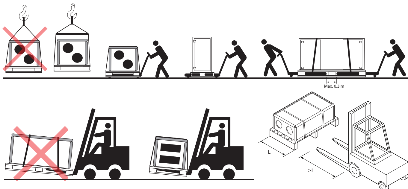
Fig. 5. Exemples de transport au moyen d'une grue, d'un chariot élévateur et d'un transpalette
