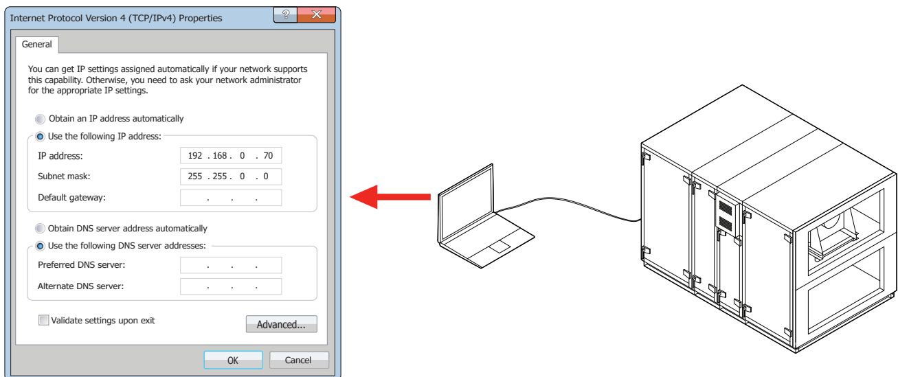
Fig. 26. Paramètres du réseau informatique pour une connexion directe à l'unité
