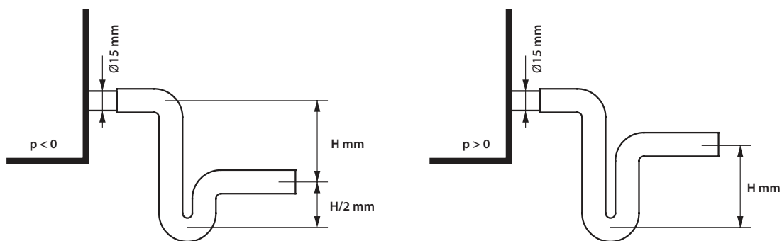
Fig. 13. Installation d'un siphon
