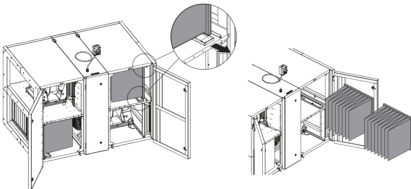
Fig. 29. Un exemple montrant comment remplacer les filtres à poches
