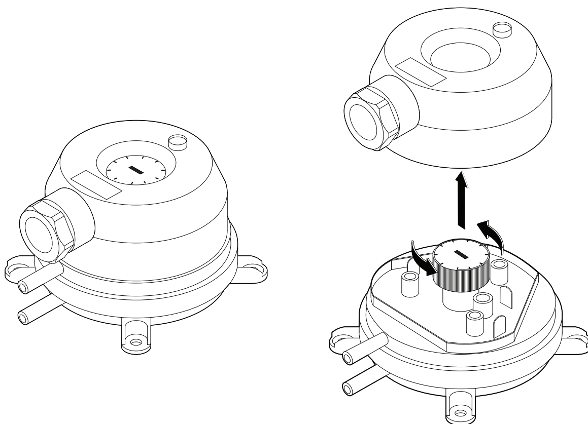
Fig. 28. Pressostat
