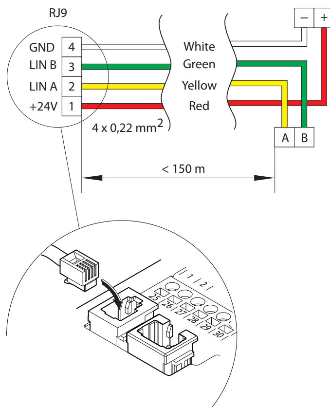
Fig. 22. Schéma de câblage du panneau de commande
